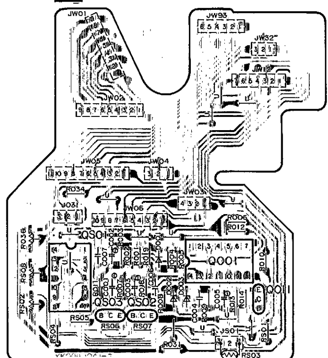
B CONNECTION P.C.B. (ZZ01D0410)
